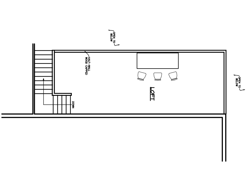
LOFT PLAN
